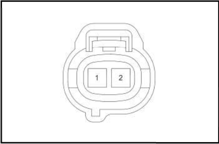
插座护套6189-0249(灰色)
