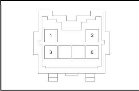
插座护套MG620401(本色)
