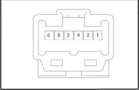
插座护套A06MW(白色)
