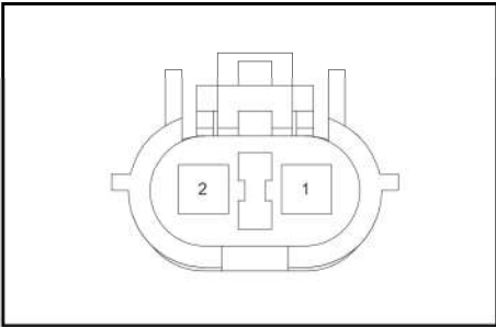
插座护套MG610320-4(灰色) 限制件MG630326-7X1
