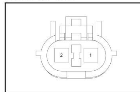
插座护套MG610320-4 (灰色)
