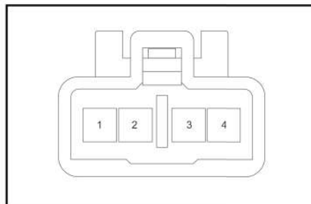
插座护套MG641041 (灰色)
